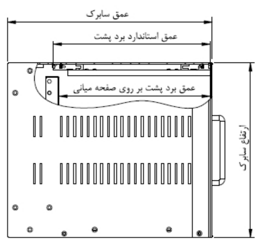
نمای کنار
