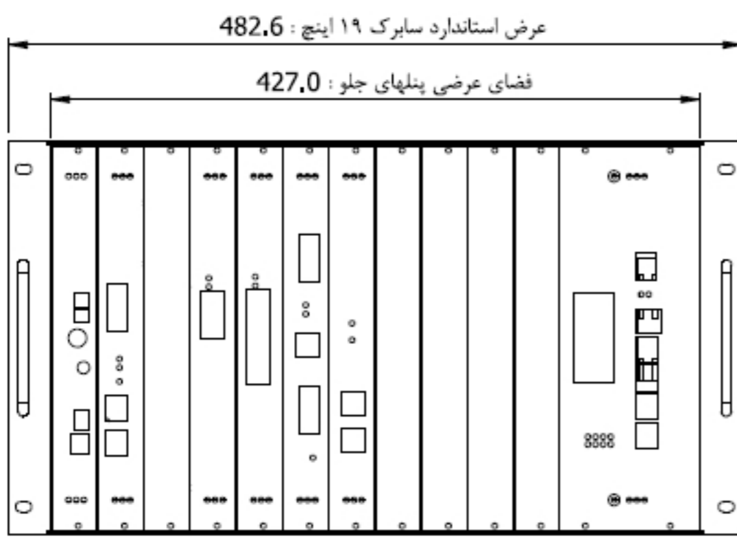
نمای روبرو
